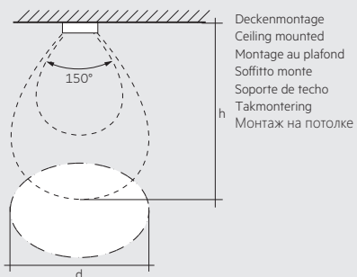
smartSWITCH HF 12DP MB f (28003498)
