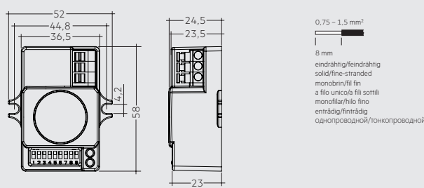
smartSWITCH HF 12DP MB S f (28003499)
