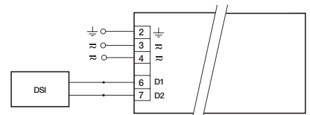
DSI PCA ECO
