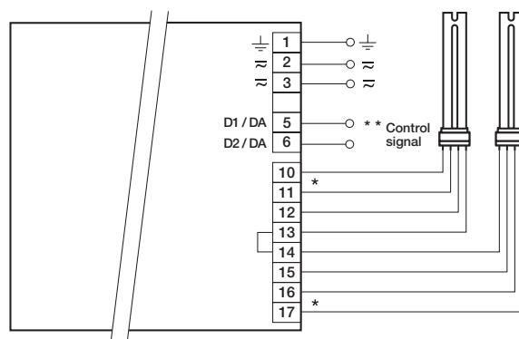
PCA TC ECO xitec II 2x18–42 W
