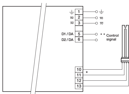
PCA TC ECO xitec II 1x18–57 W
