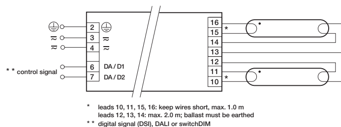
PCA T8 EXCEL one4all Ip xitec II 2x14-80 W
