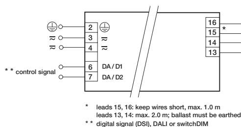
PCA T8 EXCEL one4all Ip xitec II 1x14-80 W
