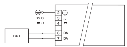
DALI PCA T8 ECO Ip xtec II
