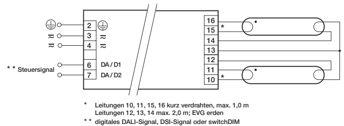
PCA T8 ECO Ip xtec II 2x14–80 W
