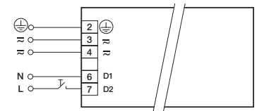
switchDIM PCA T8 ECO Ip xtec II
