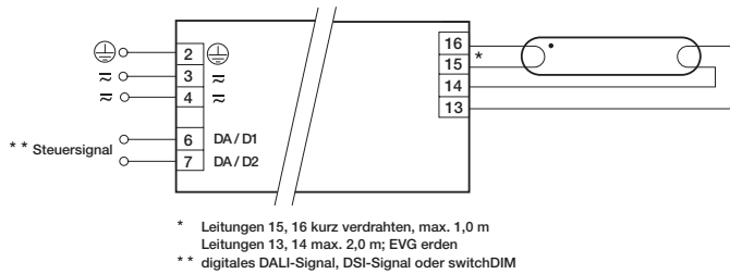
PCA T8 ECO Ip xtec II 1x14–80 W
