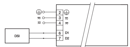
DSI PCA T8 ECO Ip xtec II
